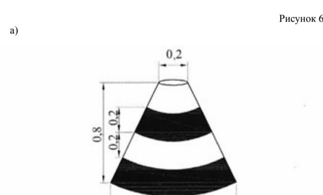
На рисунках 2, 3, 5 – 8 все размеры указаны в метрах.
