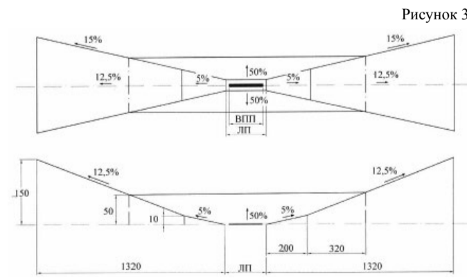
На рисунках 1 – 3 все размеры указаны в метрах.
