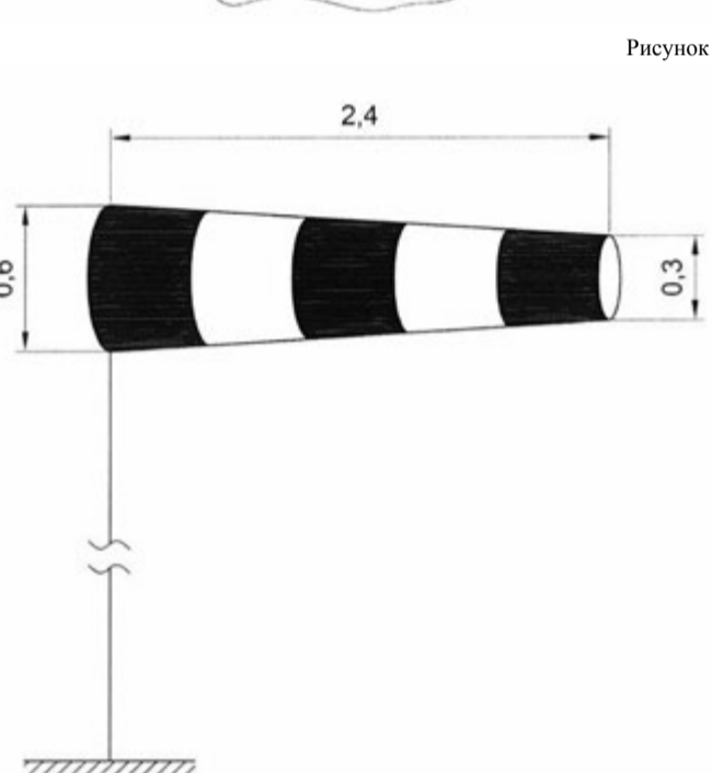
На рисунках 2, 3, 5 – 8 все размеры указаны в метрах.
